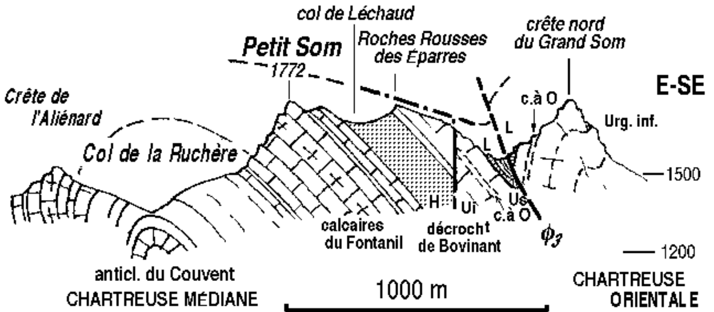
Coupe entre les crêtes de l'Aliénard et de la Dent de l'Ours
