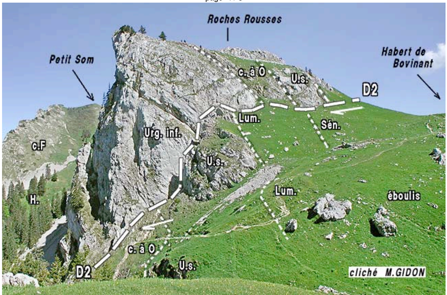
Pentes de Bovinant , vues du sud : D2 = décrochement de Bovinant.
