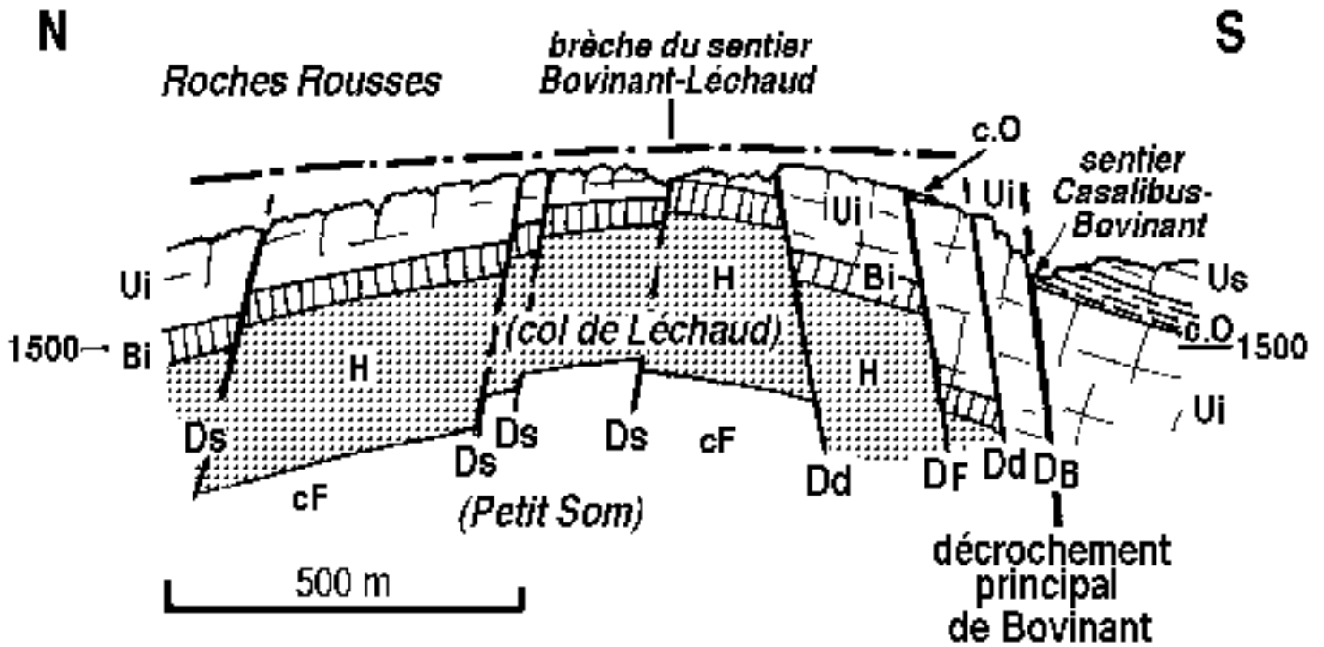
Deux vues depuis le sommet du Petit Som et la coupe correspondante
