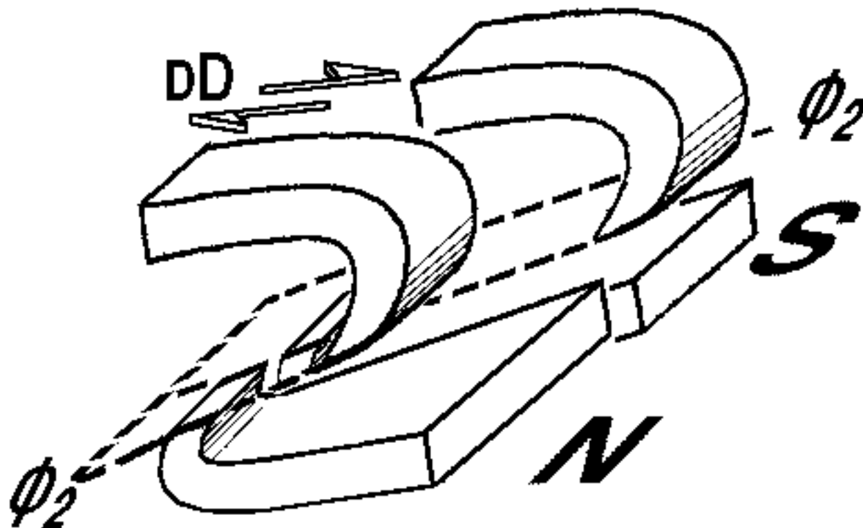
Tectonogramme très schématique des rapports décrochement - chevauchement.
