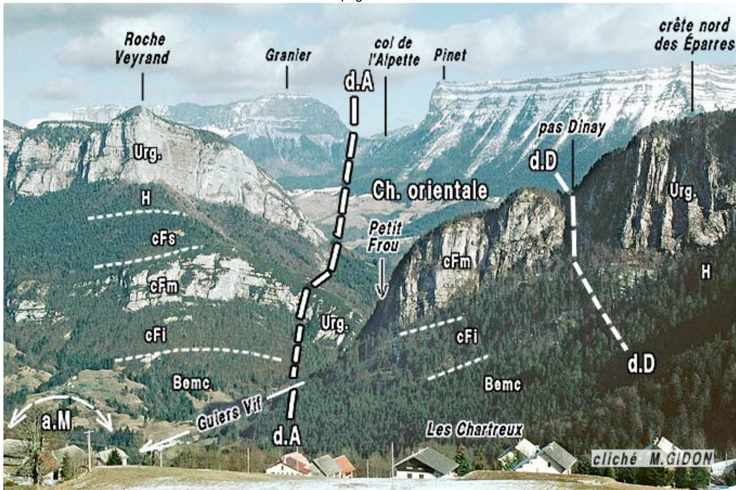
La vallée du Guiers Vif vue des pentes dominant La Ruchère (abords du foyer de ski de fond)
