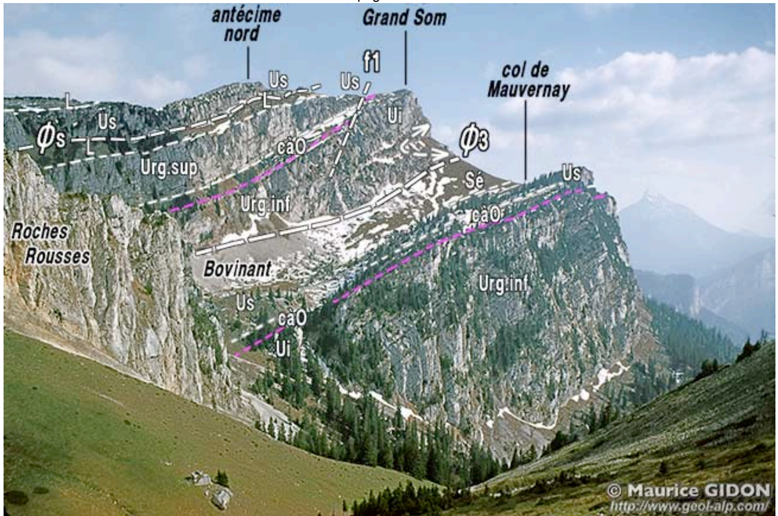
Vues sur le versant ouest de la crête du Grand Som
