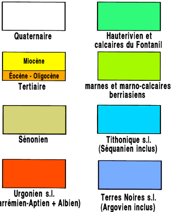
Légende de la carte géologique simplifiée de la Chartreuse
